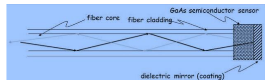
GaAsセンサー部
