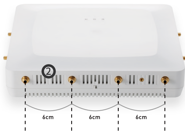
バックホール用アンテナ端子
